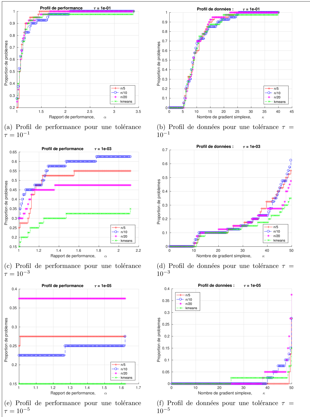
Figure 5.4 Profils de performance et de données pour des implémentations de PCA-MADS avec différentes dimensions du sous-problème (paramètre p ), sur une partie de la suite de fonctions bbob-largescale (première instance des fonctions 1 à 10) en dimension 80, 160, 320, 640 de coco avec un budget de 50n
