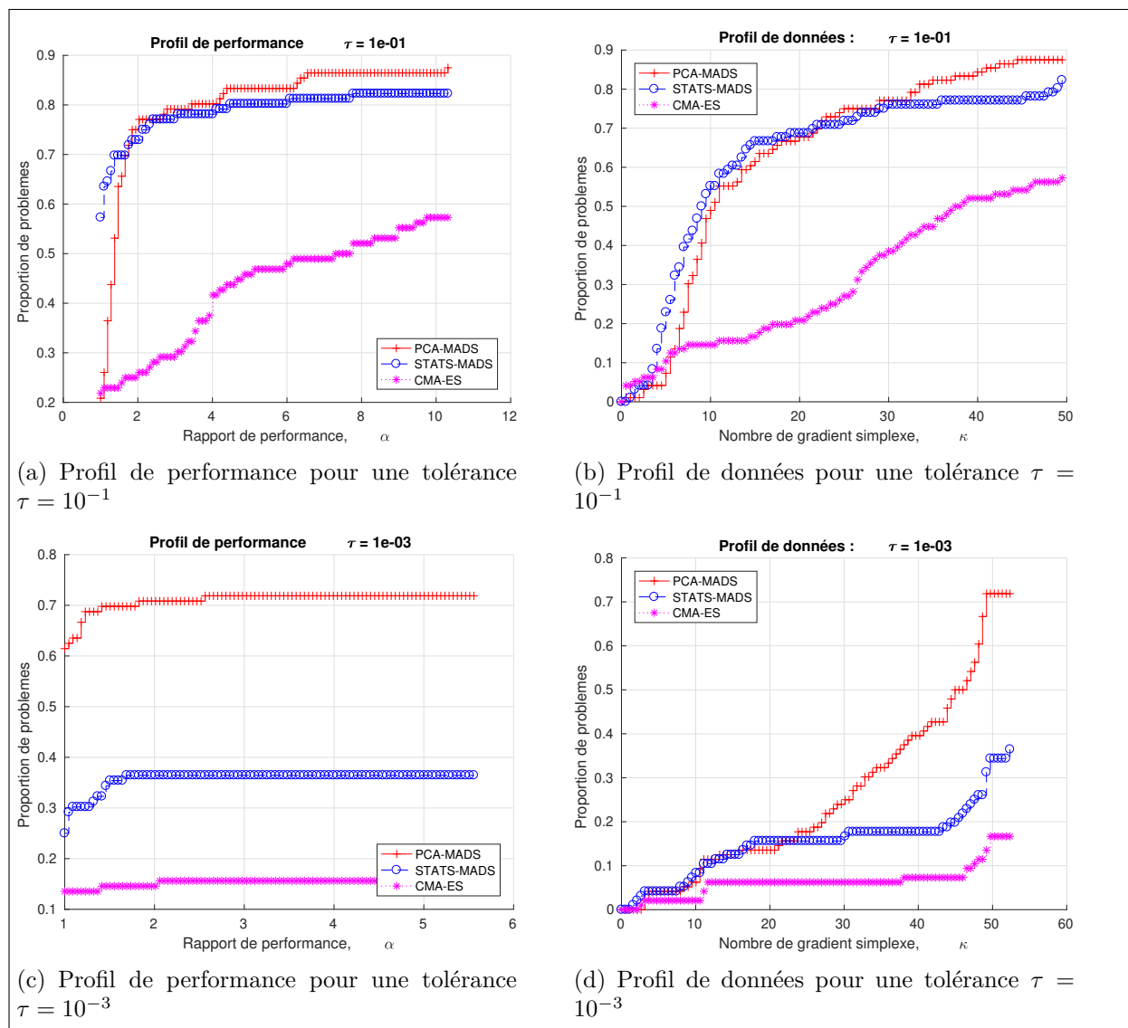
Figure 5.12 Comparaison des algorithmes PCA-MADS, STATS-MADS et CMA-ES au moyen de profils de performance et de données sur la suite de fonctions BBOB-largescale en dimension 80, 160, 320 de coco avec un budget de 50n
