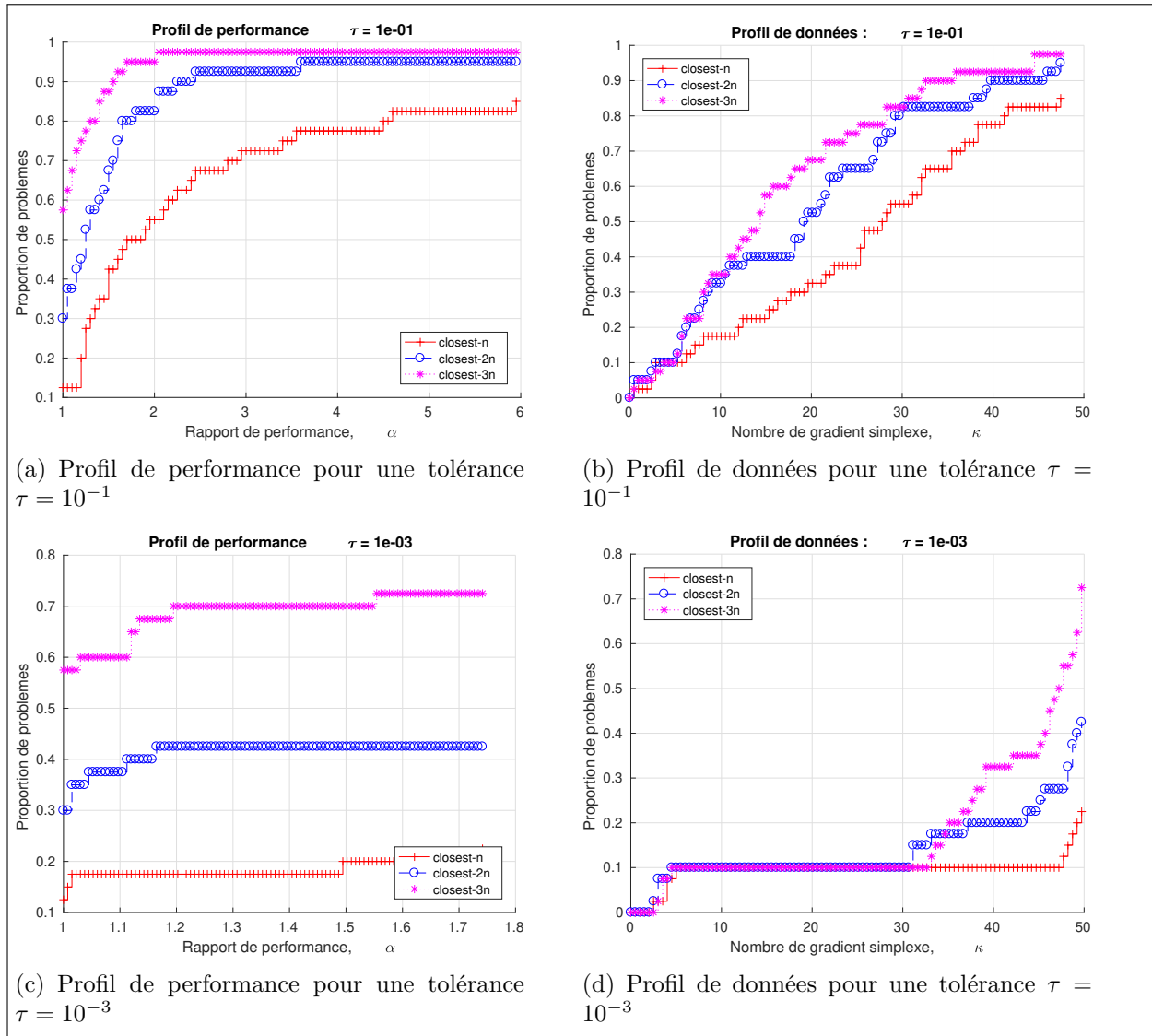
Figure 5.7 Profils de performance et de données pour des implémentations de PCA-MADS avec différents nombres des derniers points les plus proches de la solution courante pour l'analyse de sensibilité (stratégie closest - n ), sur une partie de la suite de fonctions bbob-largescale (première instance des fonctions 2, 4, 7, 9, 11, 13, 16, 18, 21 et 23) en dimension 80, 160, 320 de coco avec un budget de 50n
