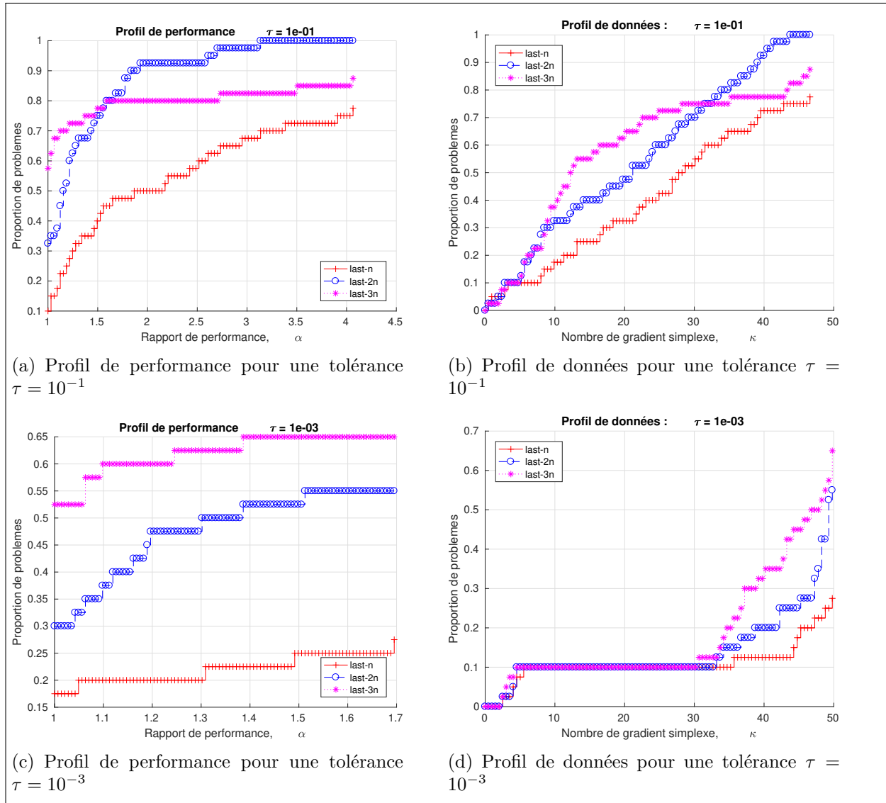
Figure 5.6 Profils de performance et de données pour des implémentations de PCA-MADS avec différents nombres des derniers points pour l'analyse de sensibilité (stratégies last-n ), sur une partie de la suite de fonctions bbob-largescale (première instance des fonctions 2, 4, 7, 9, 11, 13, 16, 18, 21 et 23) en dimension 80, 160, 320 de coco avec un budget de 50n
