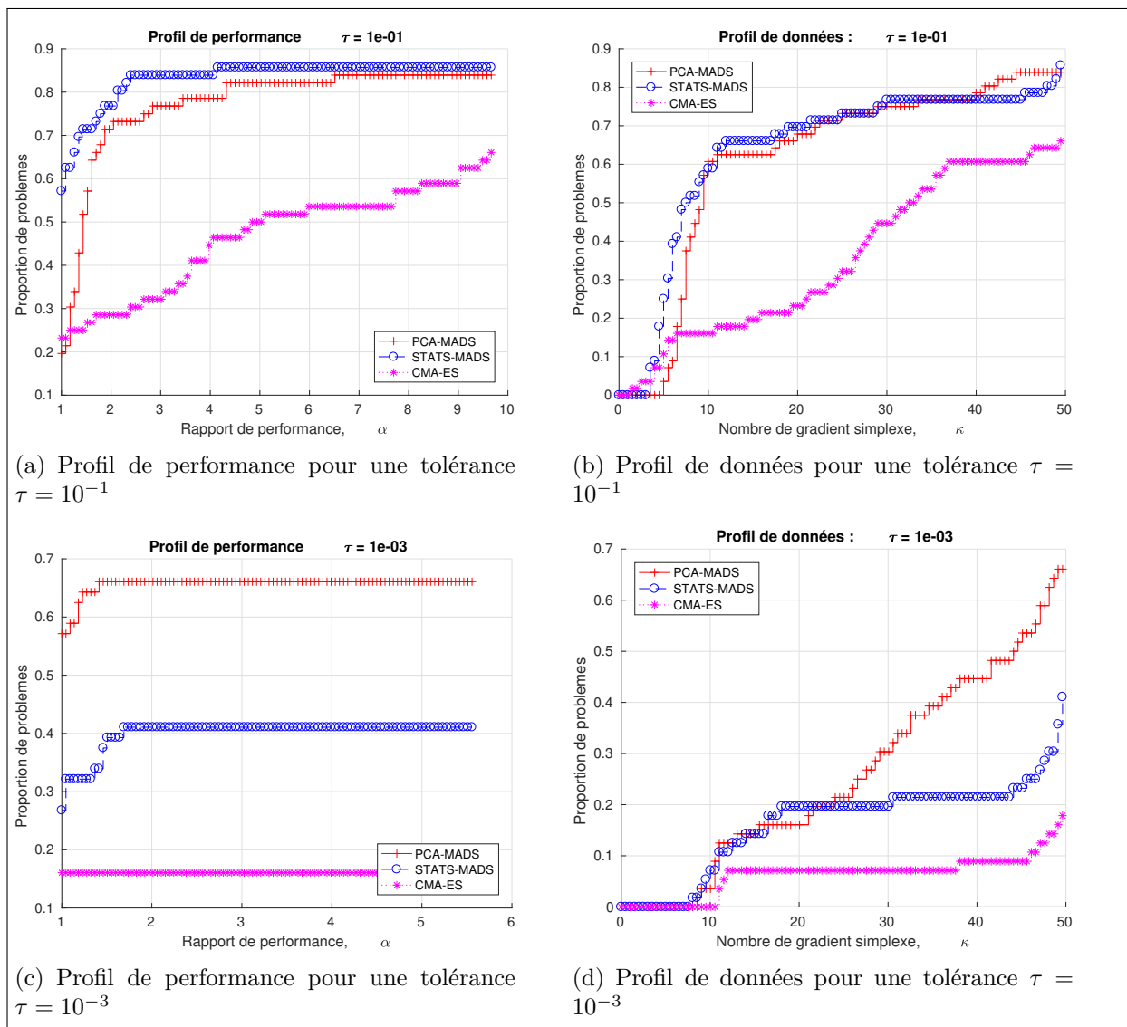
Figure 5.13 Comparaison des algorithmes PCA-MADS, STATS-MADS et CMA-ES au moyen de profils de performance et de données sur une partie de la suite de fonctions BBOB-largescale en dimension 80, 160, 320 de coco avec un budget de 50n
