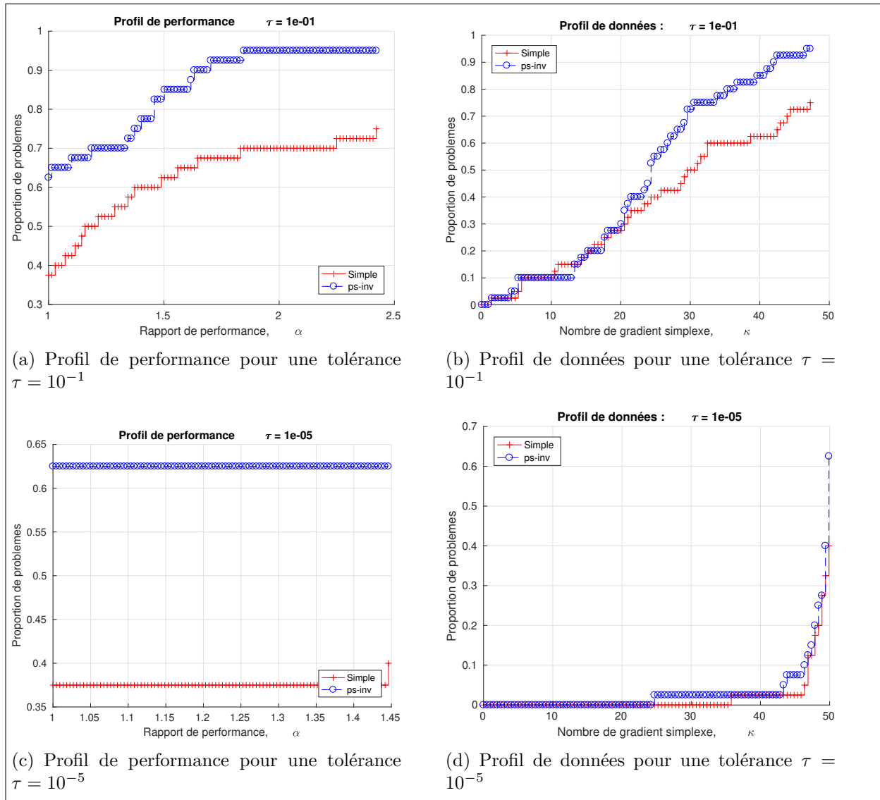
Figure 5.11 Profils de performance et de données pour des implémentations de PCA-MADS permettant de comparer les deux stratégies d'évaluation du sous-problème présentées aux équations (4.5) et (4.12), sur une partie de la suite de fonctions bbob-largescale (première instance des fonctions 2, 4, 7, 9, 11, 13, 16, 18, 21 et 23) en dimension 80, 160, 320 de coco avec un budget de 50n
