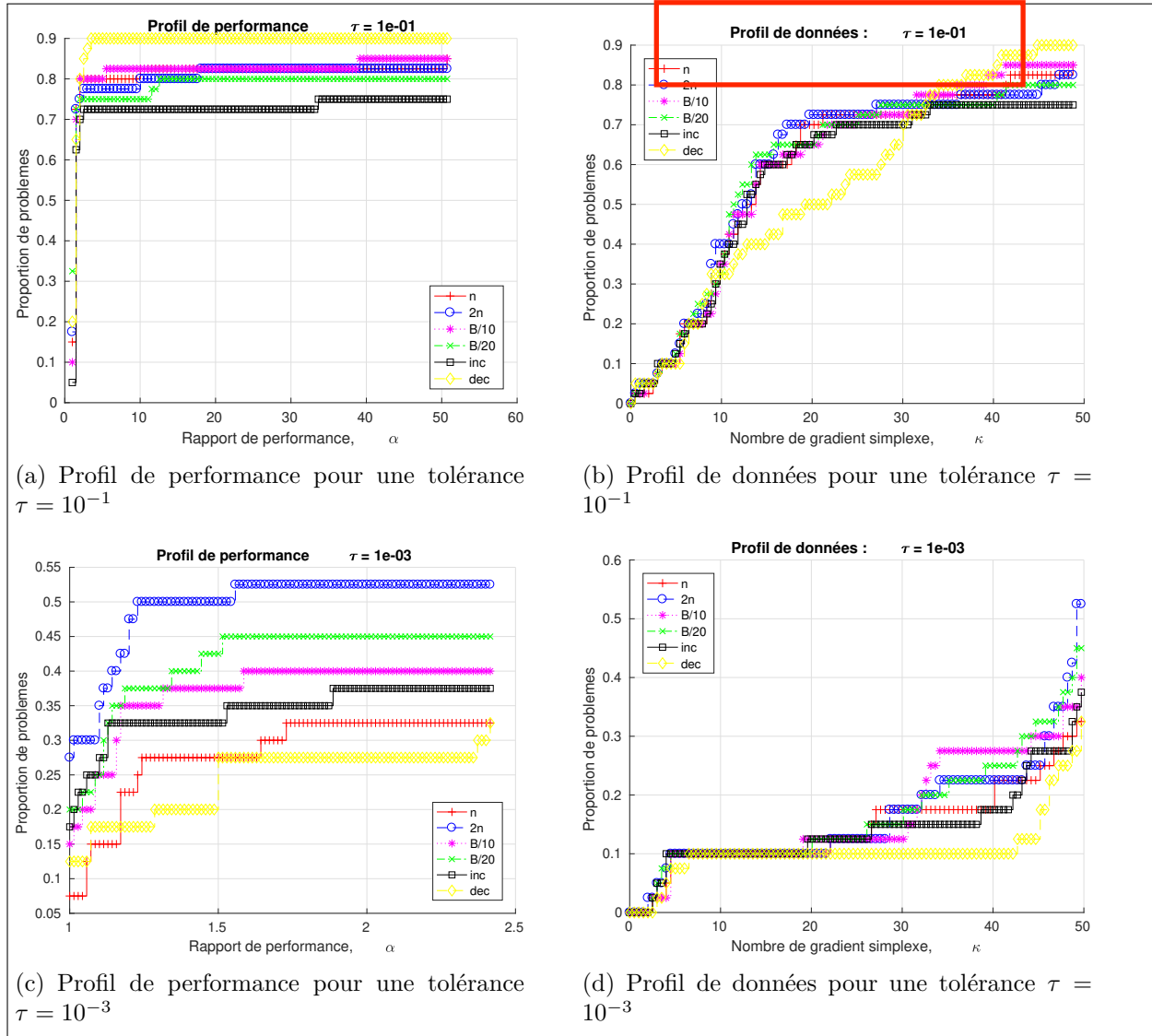
Figure 5.5 Profil de performance et de données pour des implémentations de PCA-MADS avec différents budgets d'évaluations pour l'optimisation du sous-problème, sur une partie de la suite de fonctions bbob-largescale (première instance des fonctions 2, 4, 7, 9, 11, 13, 16, 18, 21 et 23) en dimension 80, 160, 320 de coco avec un budget de 50n
