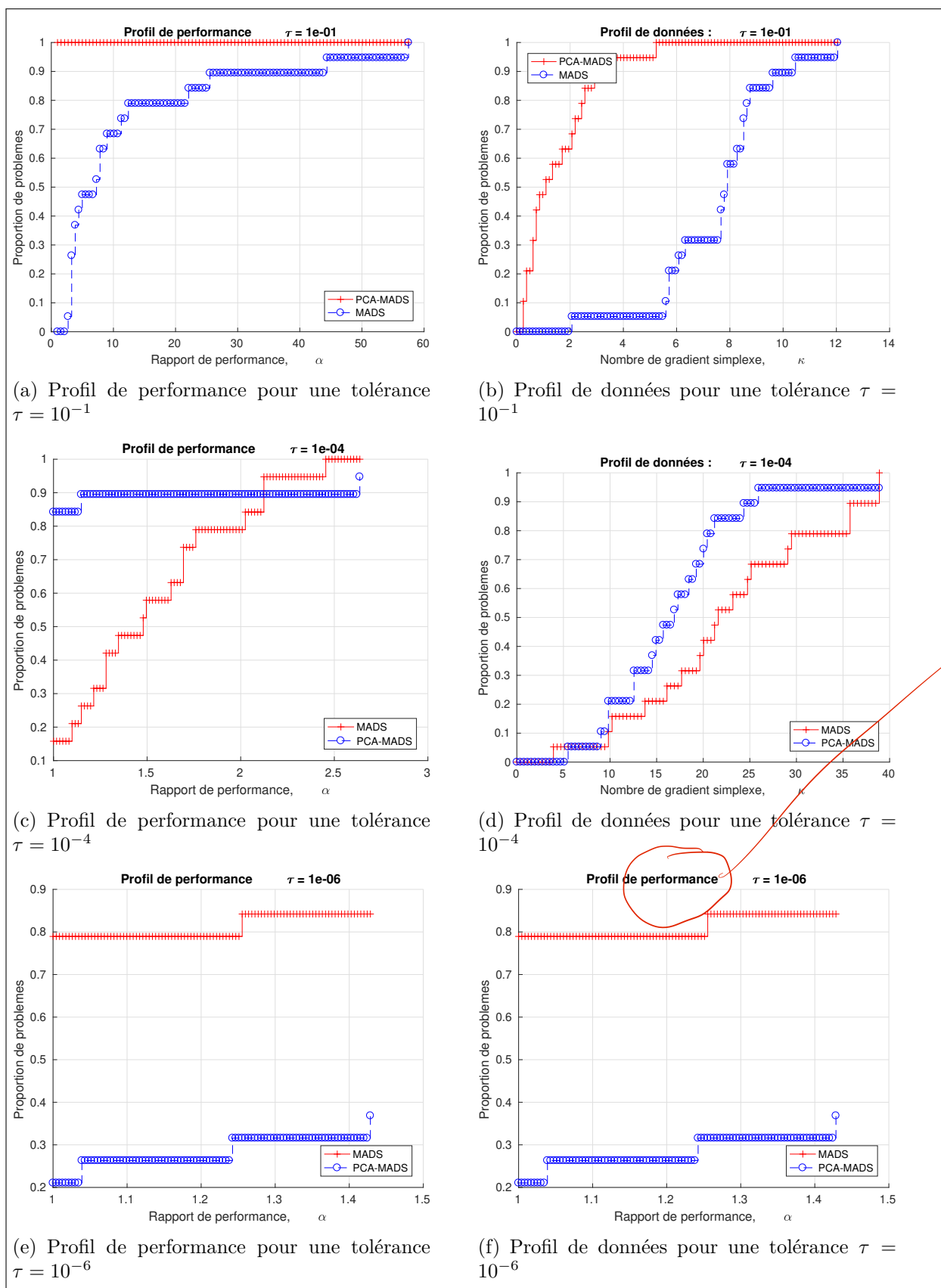
Figure 5.1 Profils de performance et de données pour un ensemble de fonctions de Rosenbrock de dimension 2, 3, 4, ..., 20 avec un budget de 100n
