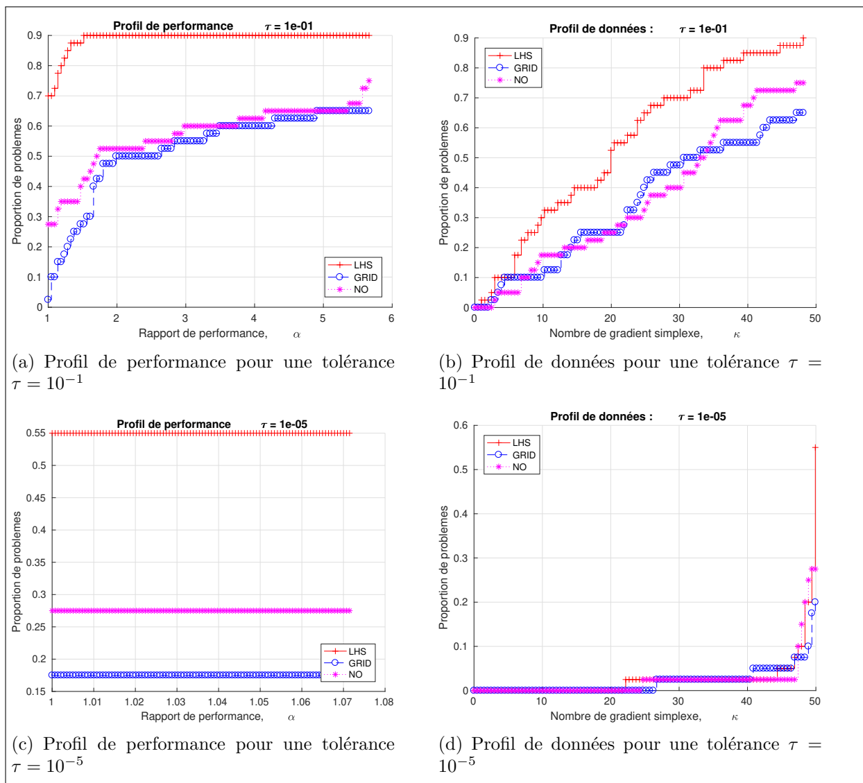
Figure 5.10 Profils de performance et de données pour des implémentations de PCA-MADS avec différentes stratégies de remplissage initial de la cache pour la première étape de recherche, sur une partie de la suite de fonctions bbob-largescale (première instance des fonctions 2, 4, 7, 9, 11, 13, 16, 18, 21 et 23) en dimension 80, 160, 320 de coco avec un budget de 50n
