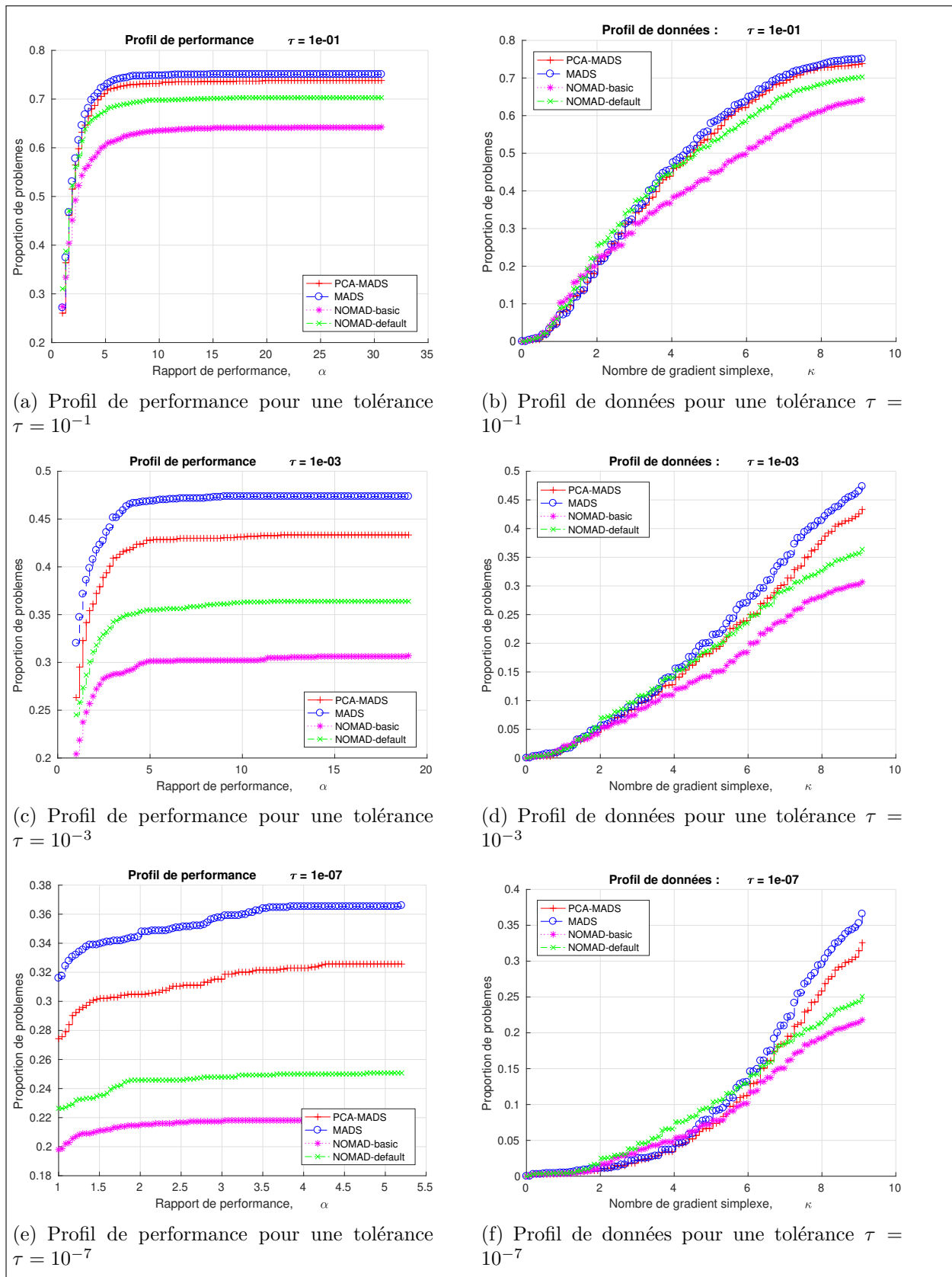
Figure 5.3 Profils de performance et de données pour des implémentations de MADS et de PCA-MADS similaire ainsi que l'implémentation NOMAD3.9.1, une version basique et la version par défaut, sur la suite de fonctions bbob de coco avec un budget de 10n
