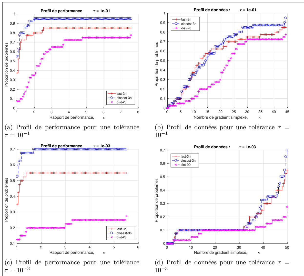
Figure 5.9 Profils de performance et de données pour des implémentations de PCA-MADS avec différentes stratégies de sélection de points pour l'analyse de sensibilité, sur une partie de la suite de fonctions bbob-largescale (première instance des fonctions 2, 4, 7, 9, 11, 13, 16, 18, 21 et 23) en dimension 80, 160, 320 de coco avec un budget de 50n
