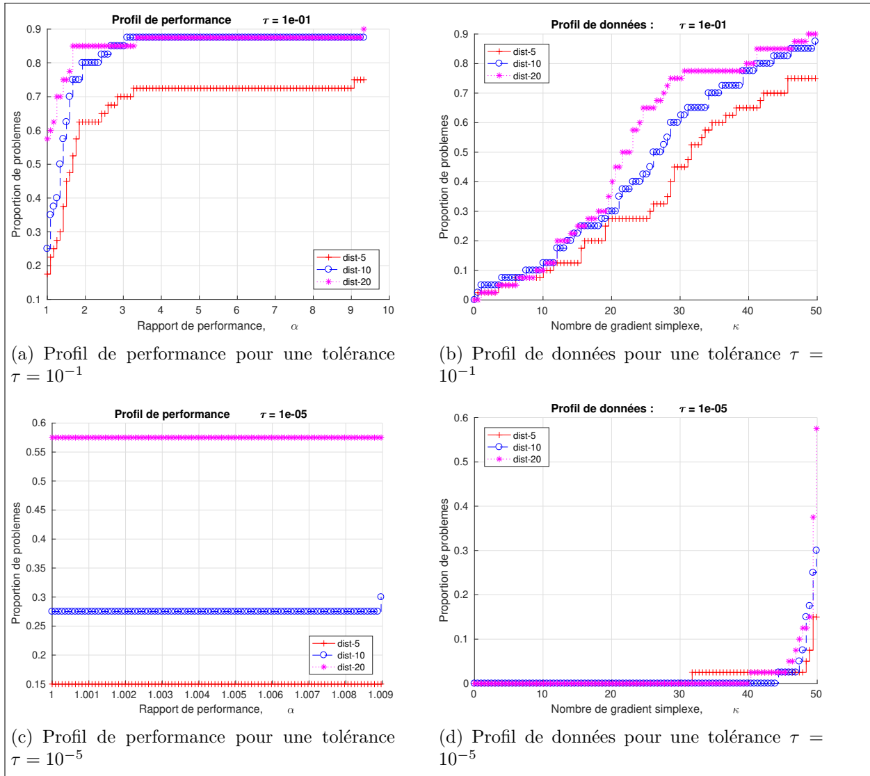
Figure 5.8 Profils de performance et de données pour des implémentations de PCA-MADS avec une stratégie de sélection de points pour l'analyse de sensibilité basée sur la distance autour de la solution courante (stratégie dist - \epsilon ), sur une partie de la suite de fonctions bbob-largescale (première instance des fonctions 2, 4, 7, 9, 11, 13, 16, 18, 21 et 23) en dimension 80, 160, 320 de coco avec un budget de 50n
